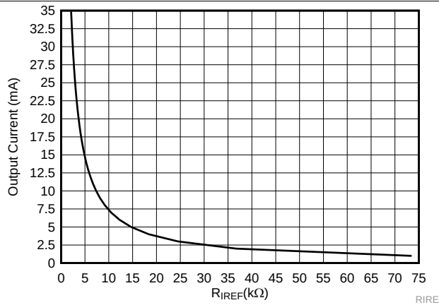
图 2. I_{OUT} Target vs R_{IREF}
