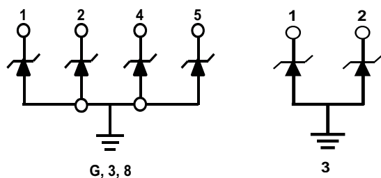
0802/1004 DFN array
