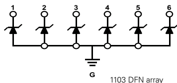
1103 DFN array
