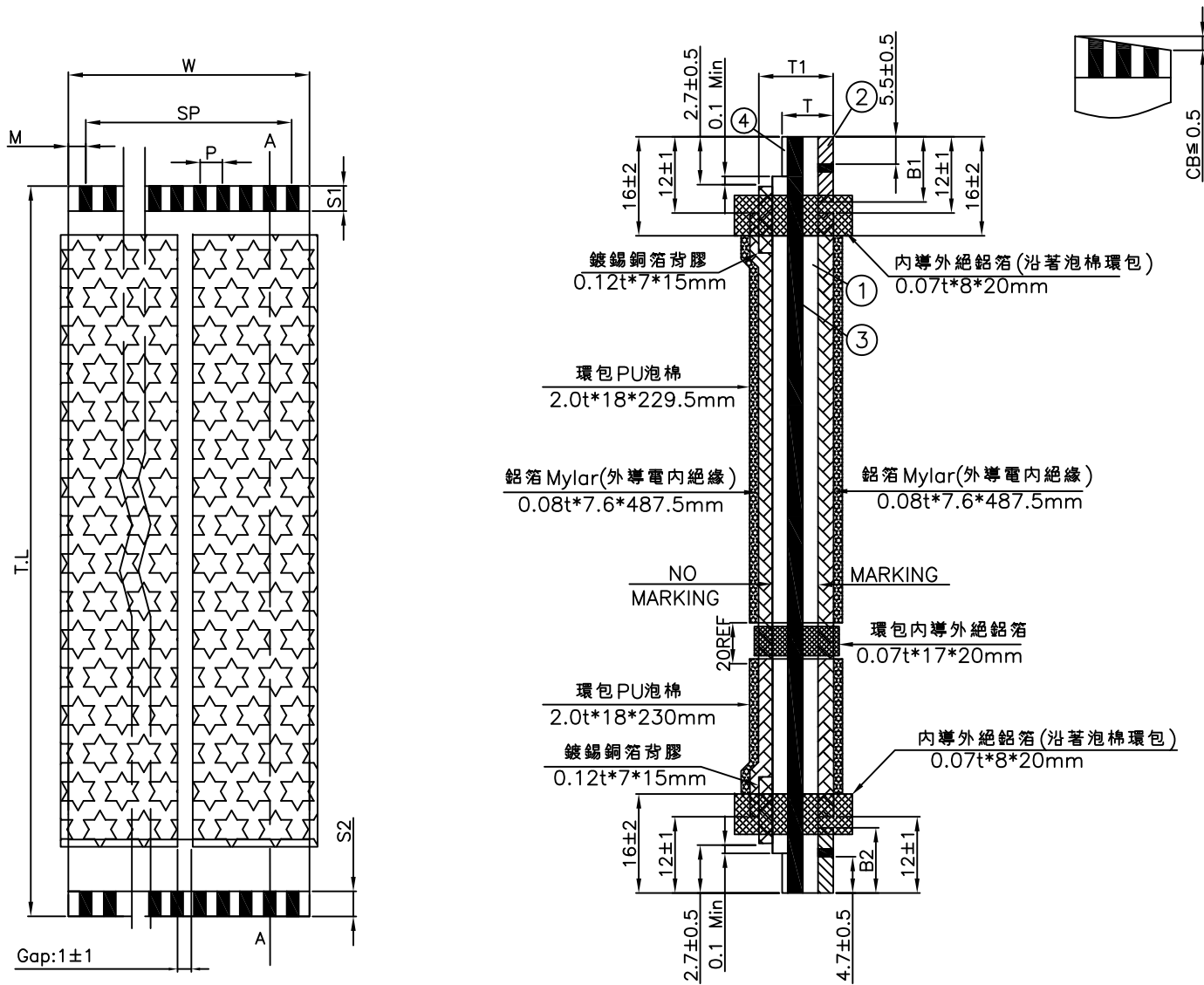
SECTION A-A
